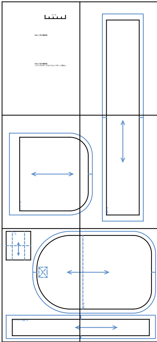
生地 1 枚の裁断図 W:520mm L:1070mm
